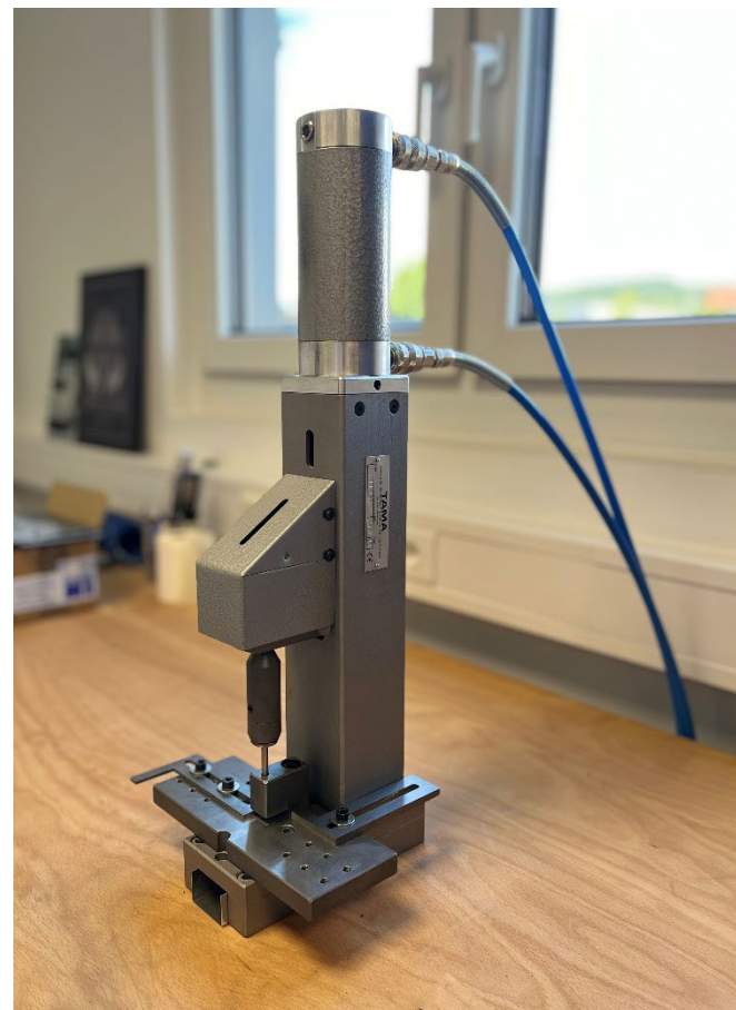
Druckluftbetriebene Stanze
